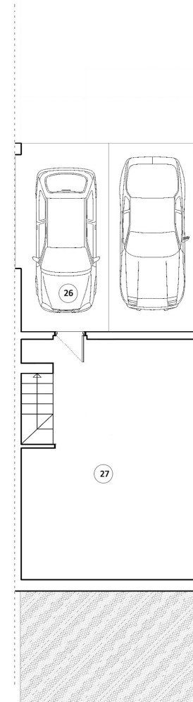
planta sótano
