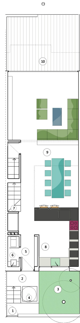
planta baja
